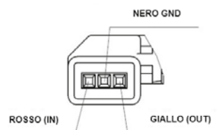
FOTO CONNETTORE PWM
